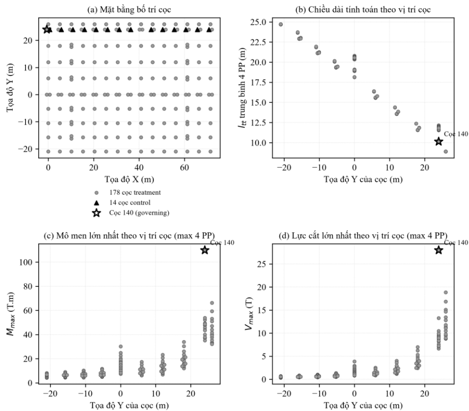
Hình 4. Phân bố không gian của độ nhảy trên 178 cọc treatment**: (a) mặt bằng bố trí cọc, đánh dấu cọc governing (140); (b) chiều dài tính toán trung bình (4 phương pháp) theo vị trí cọc; (c) mô men lớn nhất và (d) lực cắt lớn nhất (giá trị lớn nhất trong 4 phương pháp) theo vị trí cọc — cho thấy độ nhảy tập trung rõ rệt tại hàng cọc biên.
